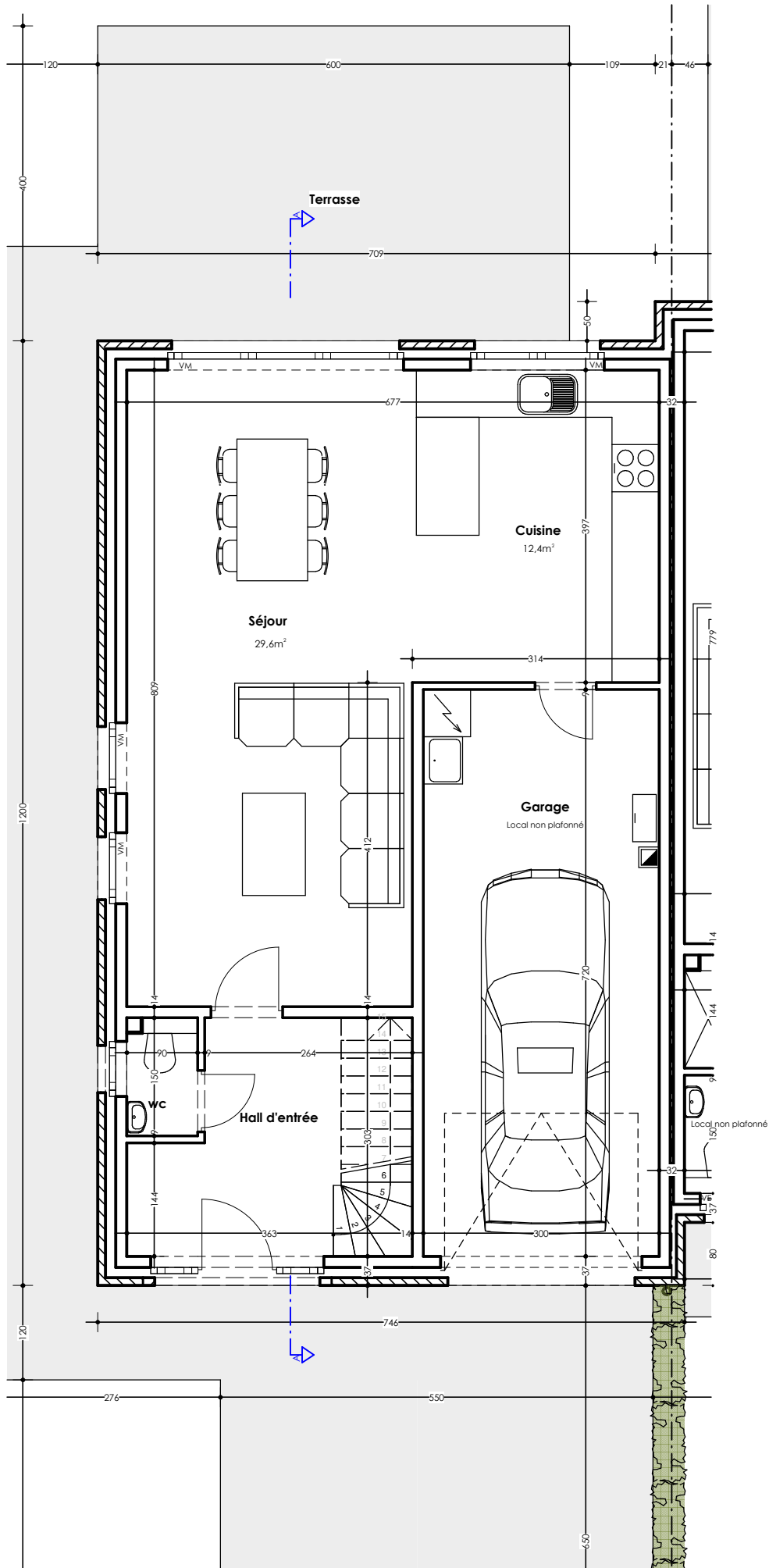
Maison 74 : Plan rez-de-chaussée
