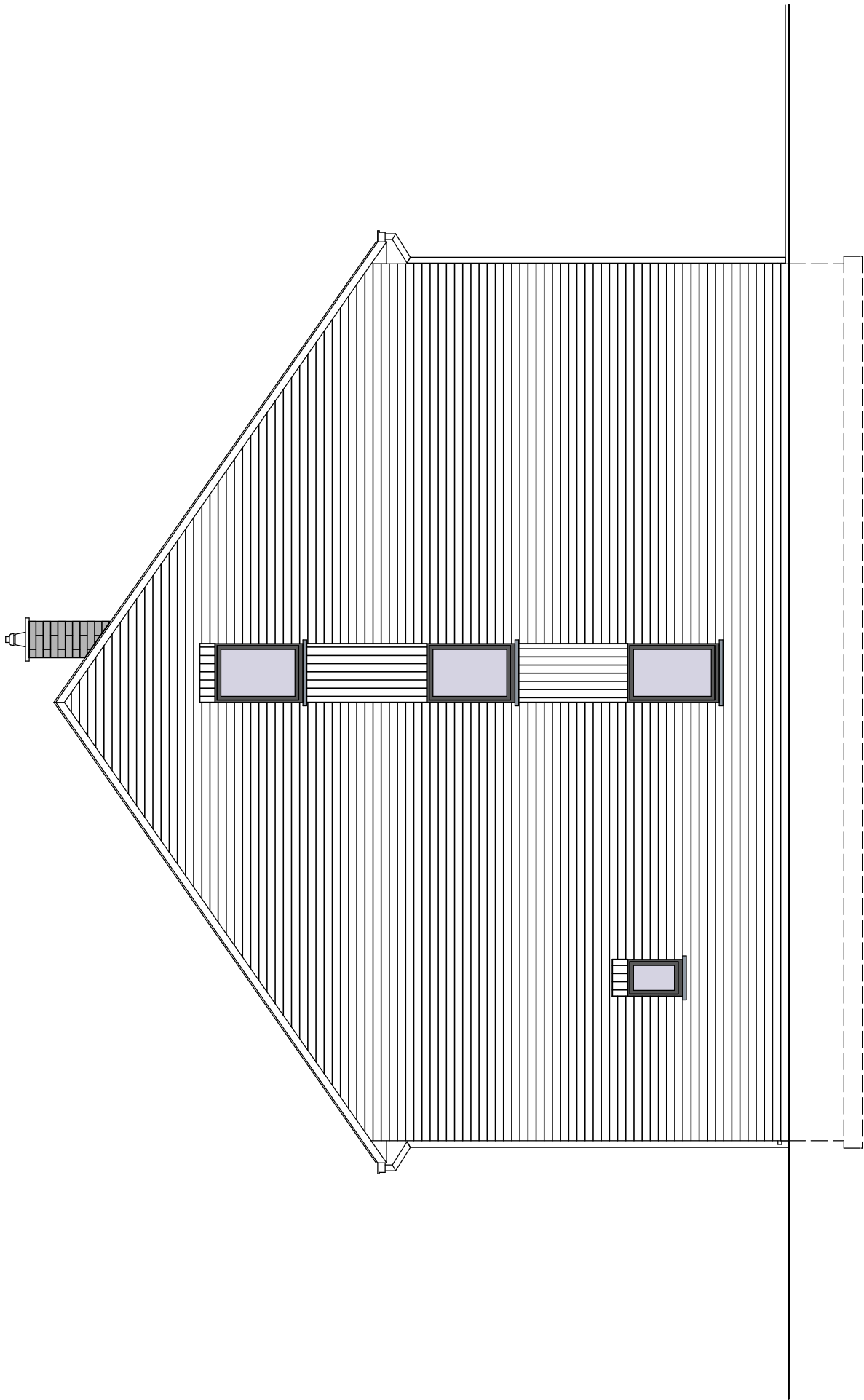
Maison 13 Façade Latérale Droite
