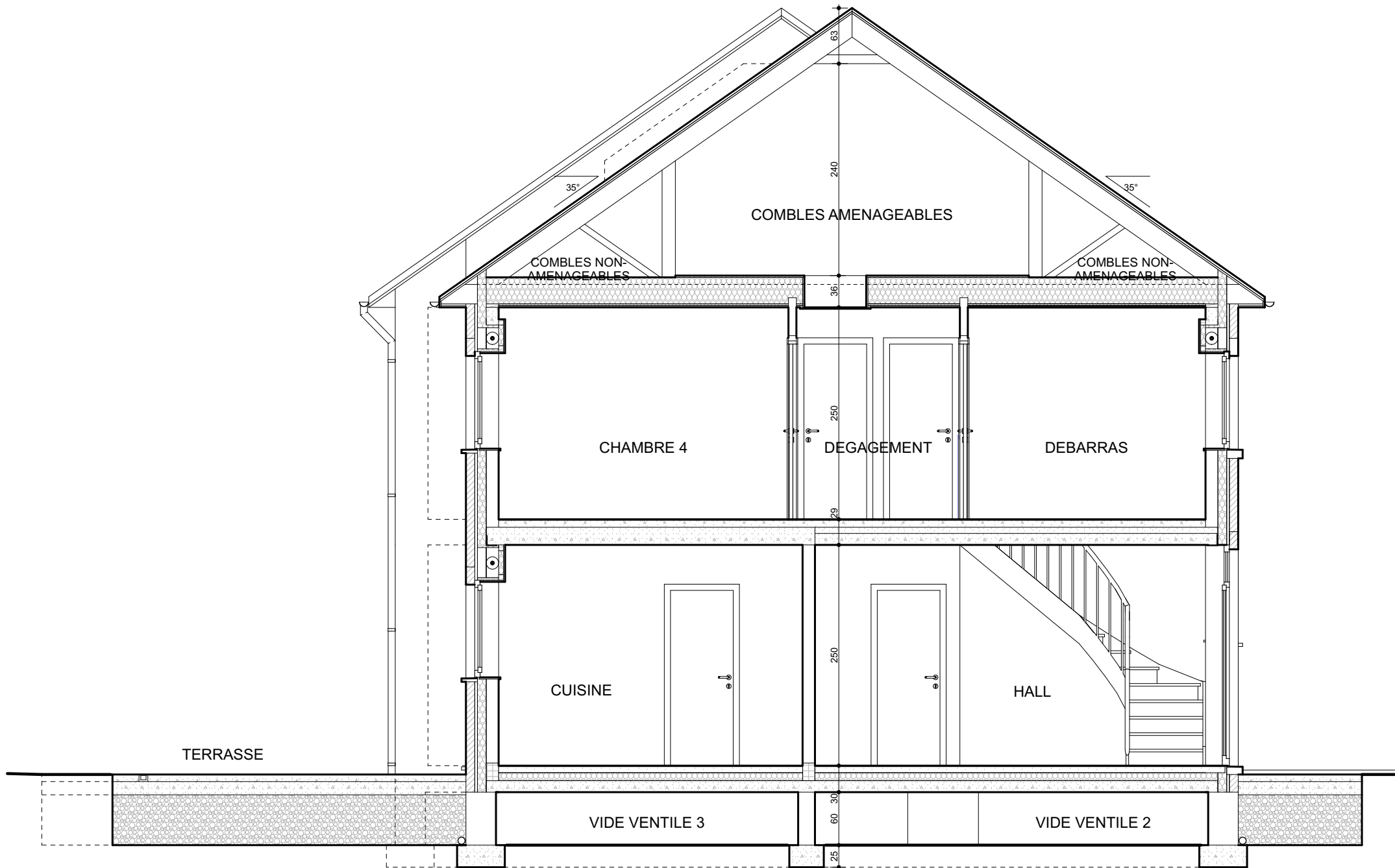
Dison : Rue du Bois des Haies Coupe AA lot 1
