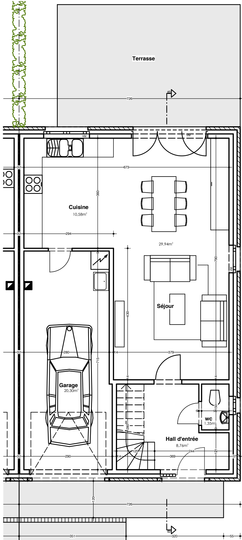
Maison 9 : Plan Rez-de-chaussée
