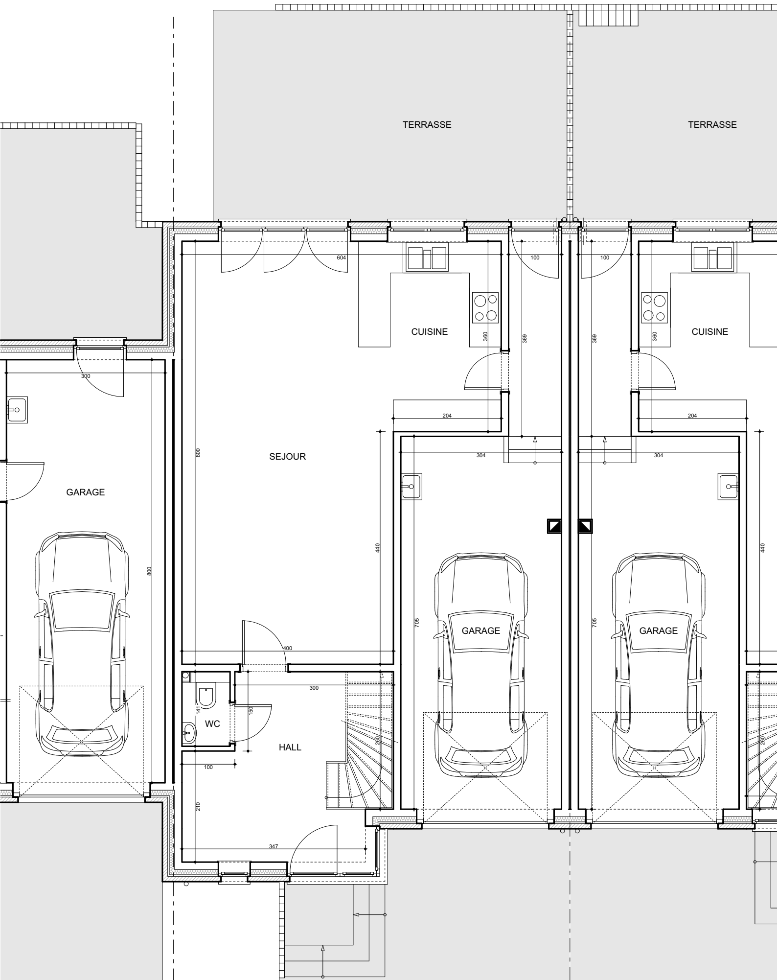
Petit-Rechain Rez-de-chaussée lot 11
