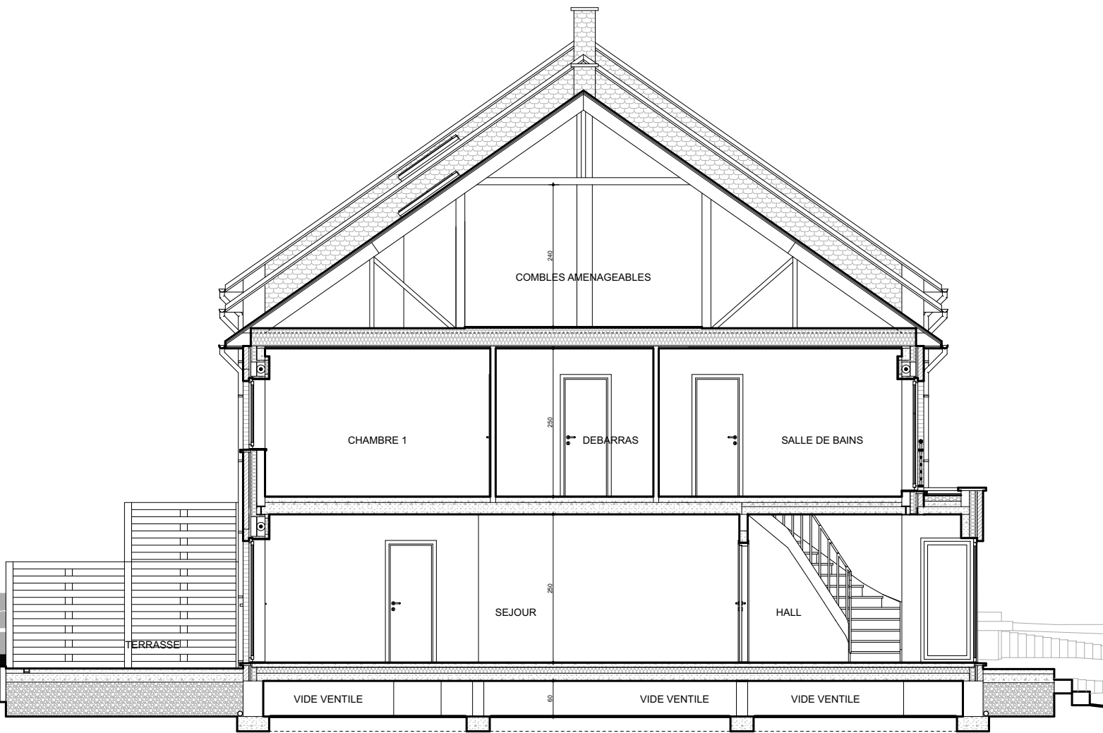
Petit-Rechain : Coupe DD lot 10
