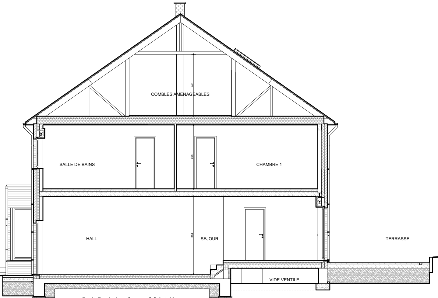
Petit-Rechain : Coupe GG lot 10
