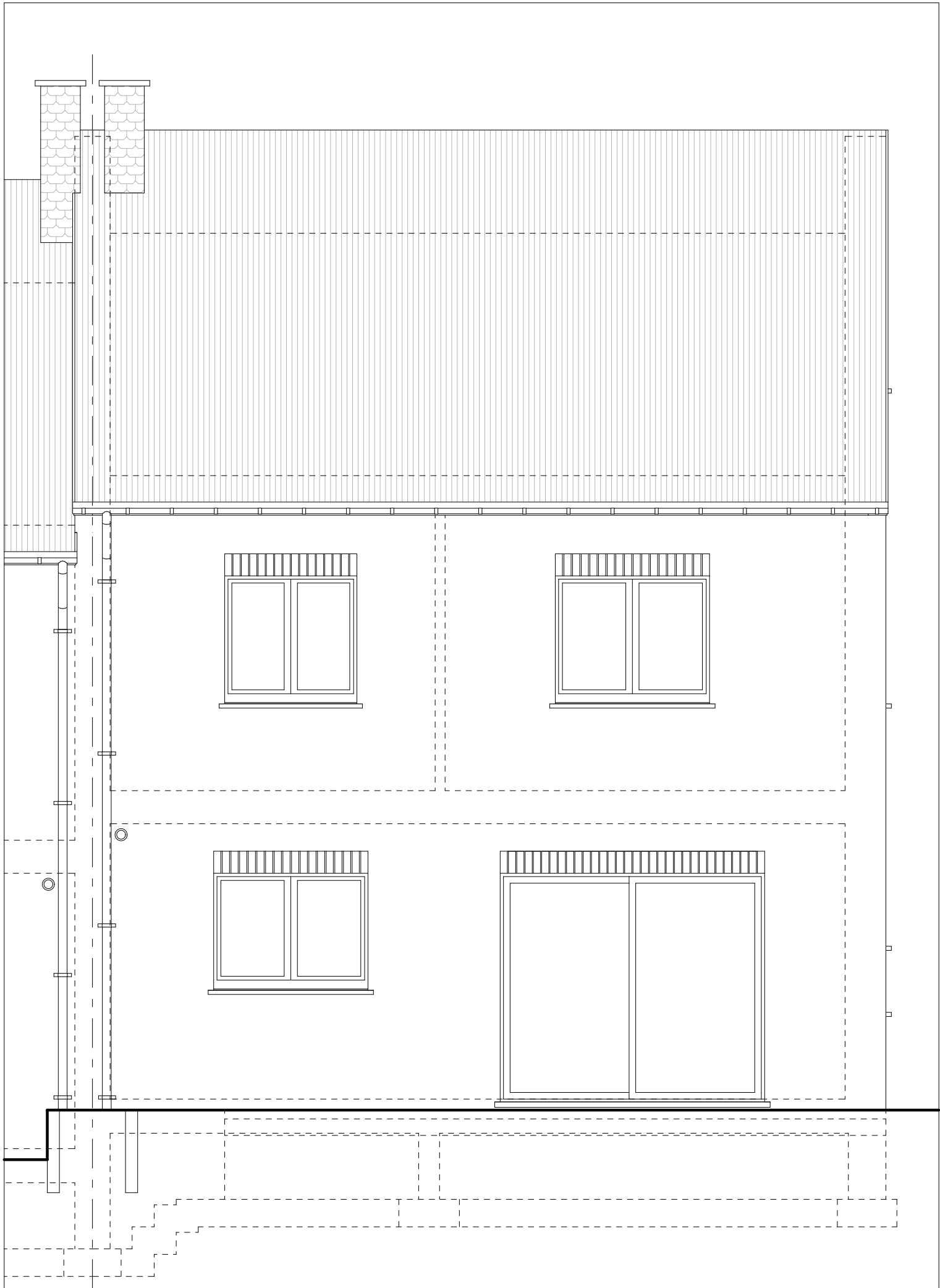
Petit - Rechain : Façade arrière lot 15
