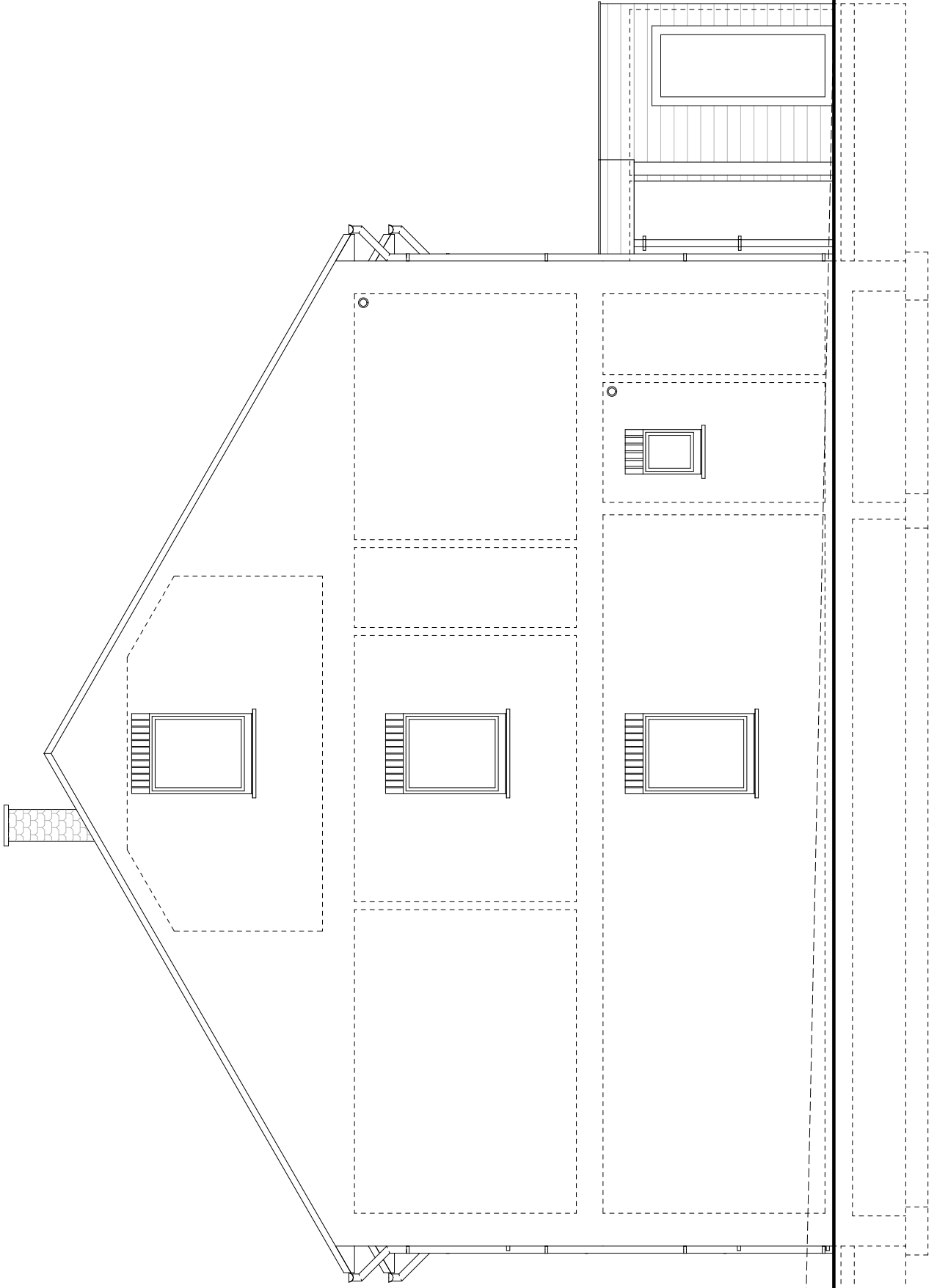
Petit - Rechain : Façade latérale gauche lot 15
