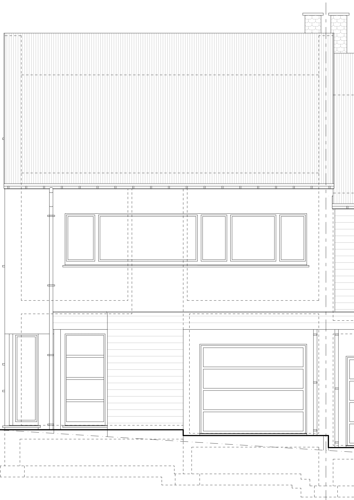
Petit - Rechain : Façade principale à rue lot 15
